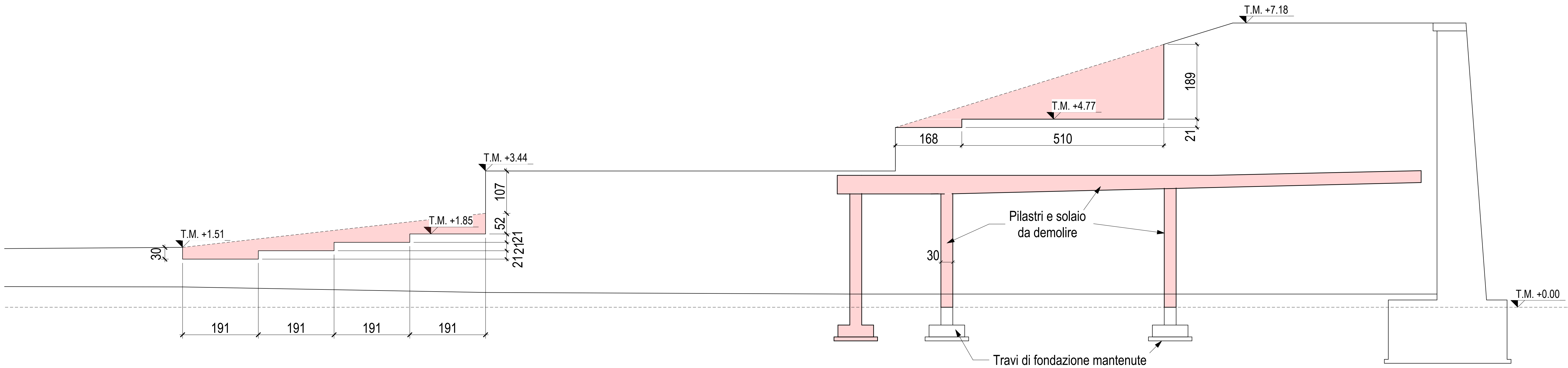
Prospetto demolizioni scala 1:50
